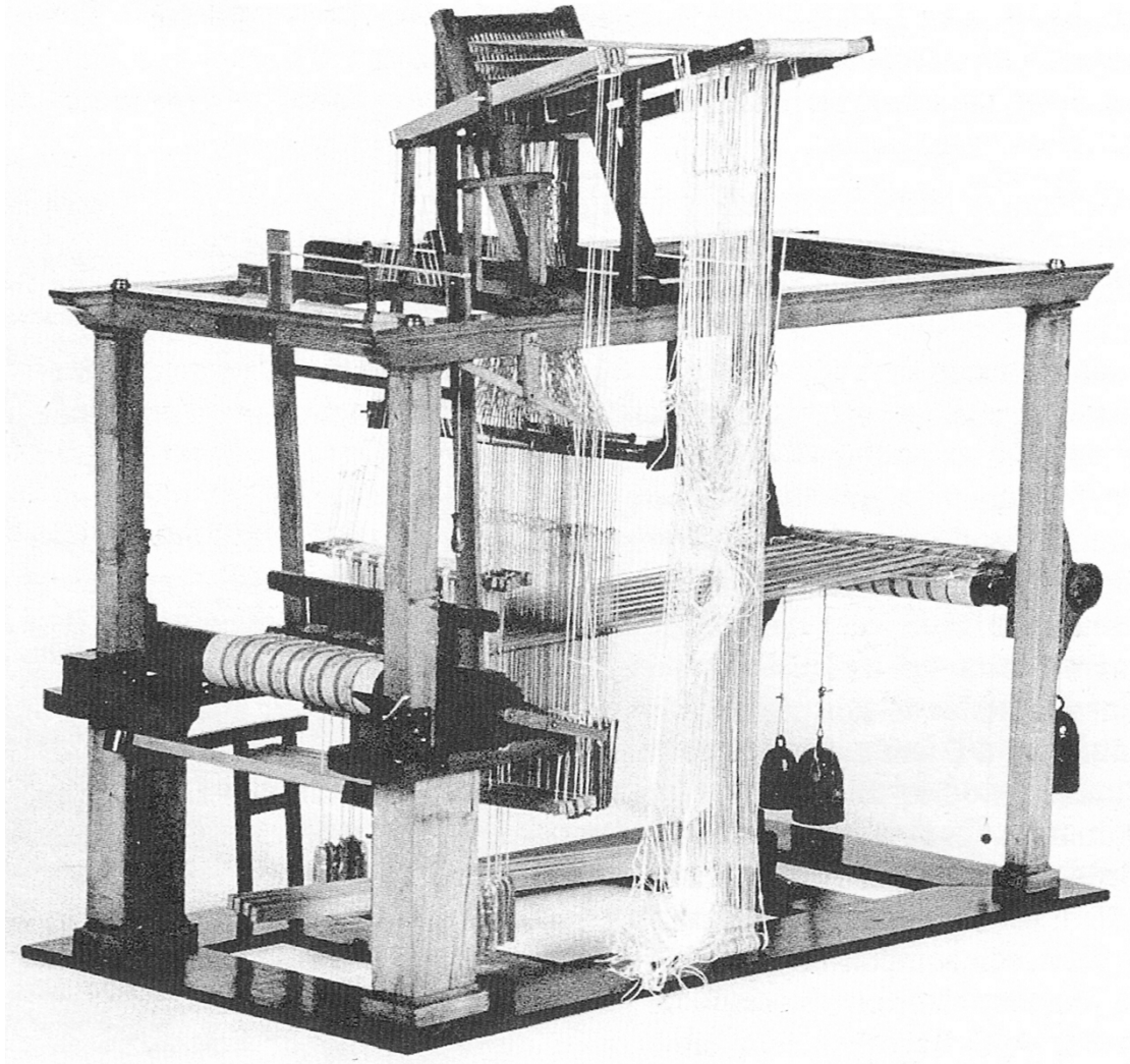
図 2：大型紋織機 métier à la grande tire （模型）
